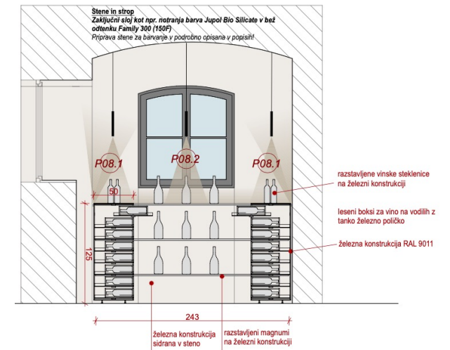
PREČNI PREZ 1'-1'
